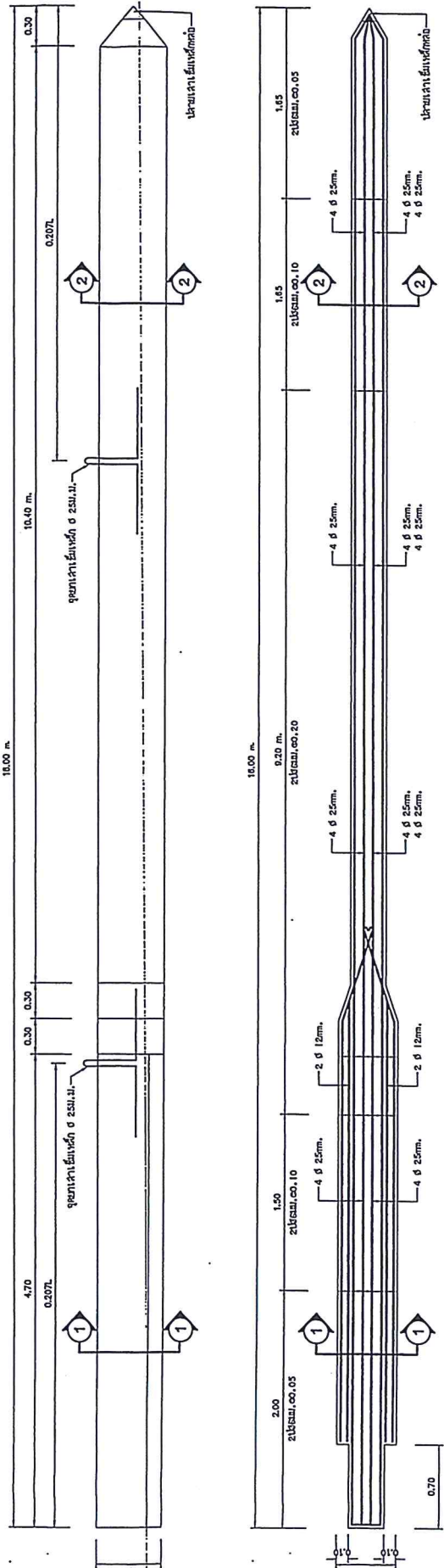
แบบรายละเอียดเสาเข็มคอนกรีตอัดแรงขนาด 0.55x0.50x16.00 ม.
